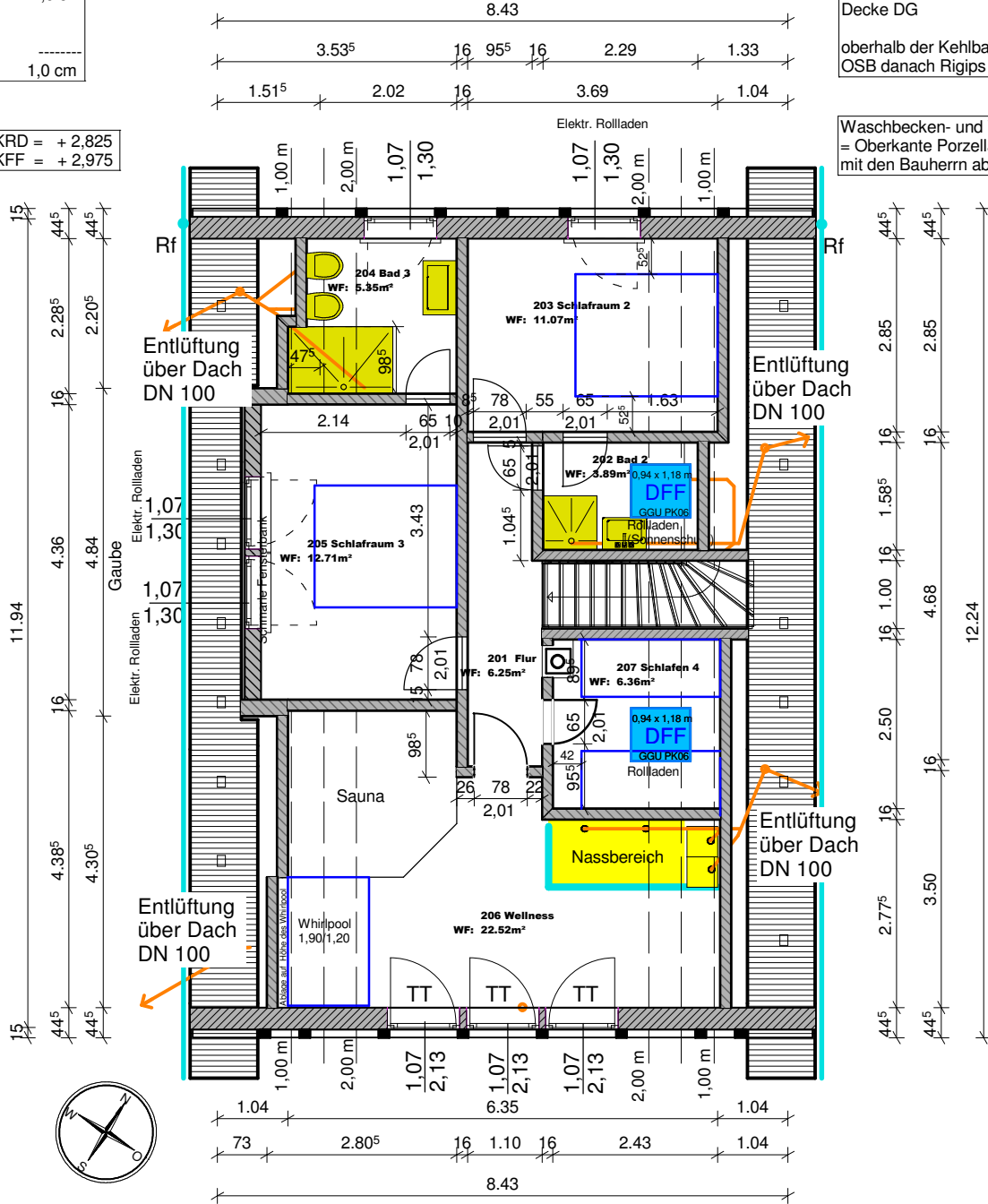
Dachgeschoss mit Entwässerung
